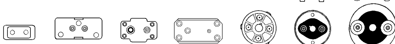
G 9.5 GX 9.5 GY 9.5 GY 16 GY 17q G 22 PG 38
